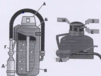
Огнетушитель воздушно-пенный
