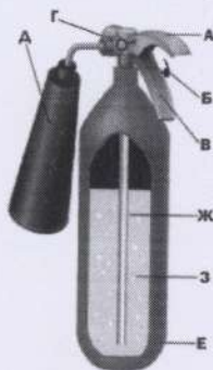
Огнетушитель углекислотный
